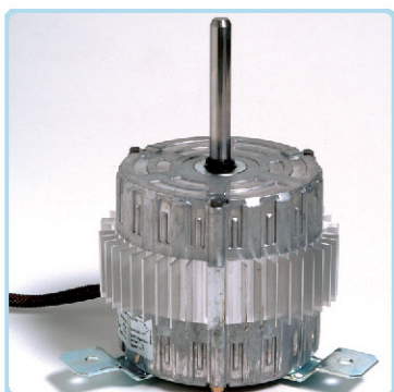
מנועי מעבה כולל צלעות קחר
