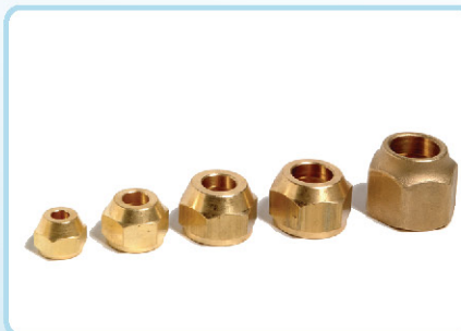
אומי פלר 3/16" - 7/8" (חישול או חריטה)
