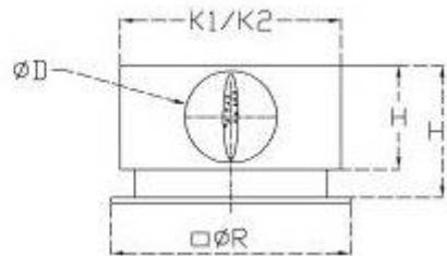
קופסת פיזור עם כניסה צידית SLT 4W-S
